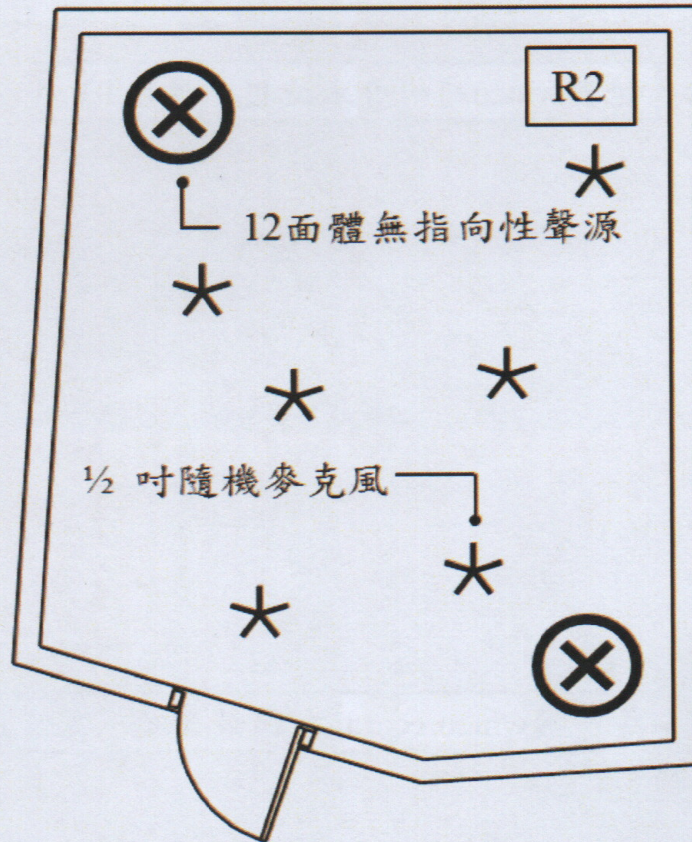
圖4.1 試驗設備配置平面示意圖
