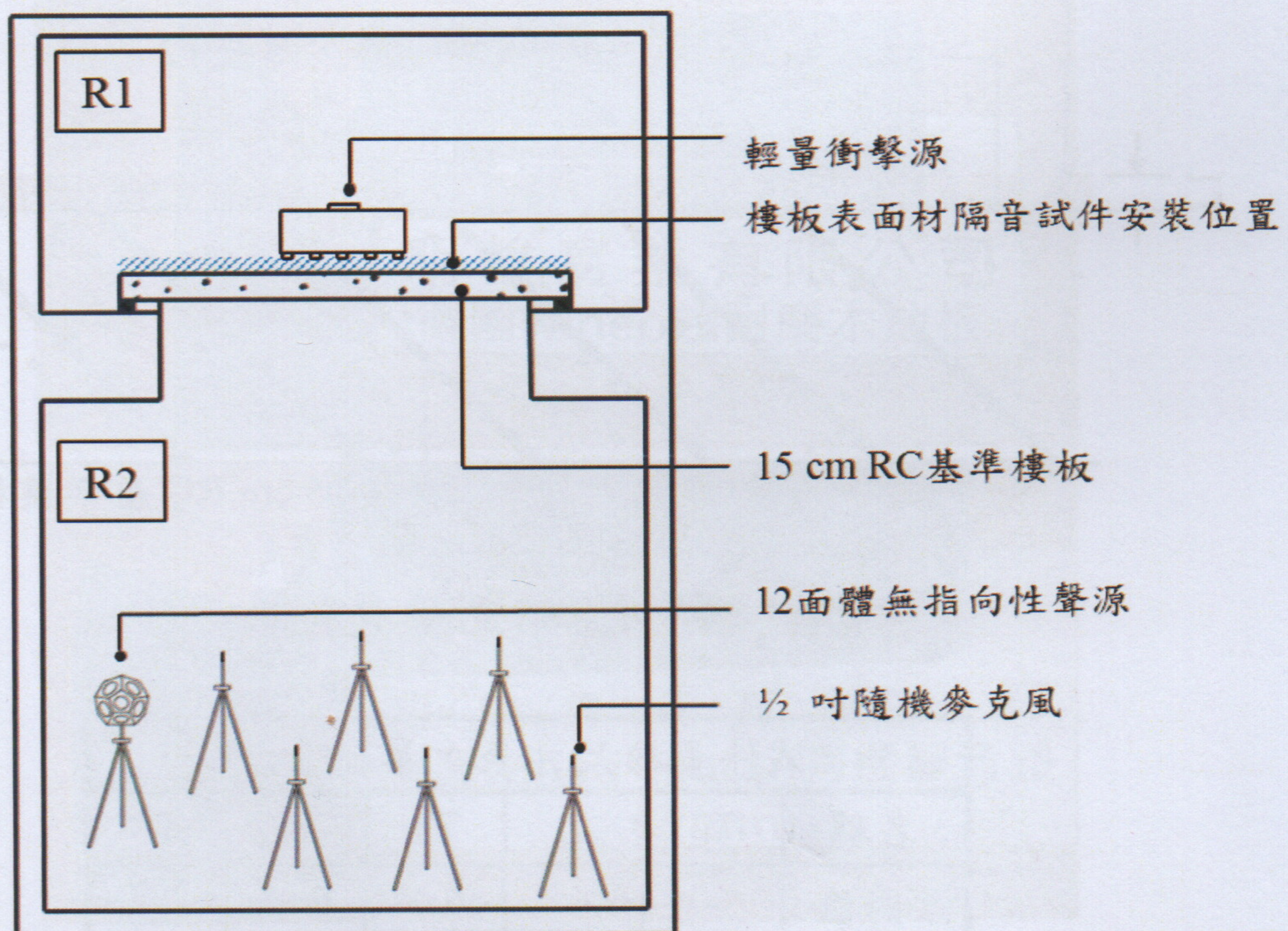
圖4.2 試驗設備配置剖面示意圖
