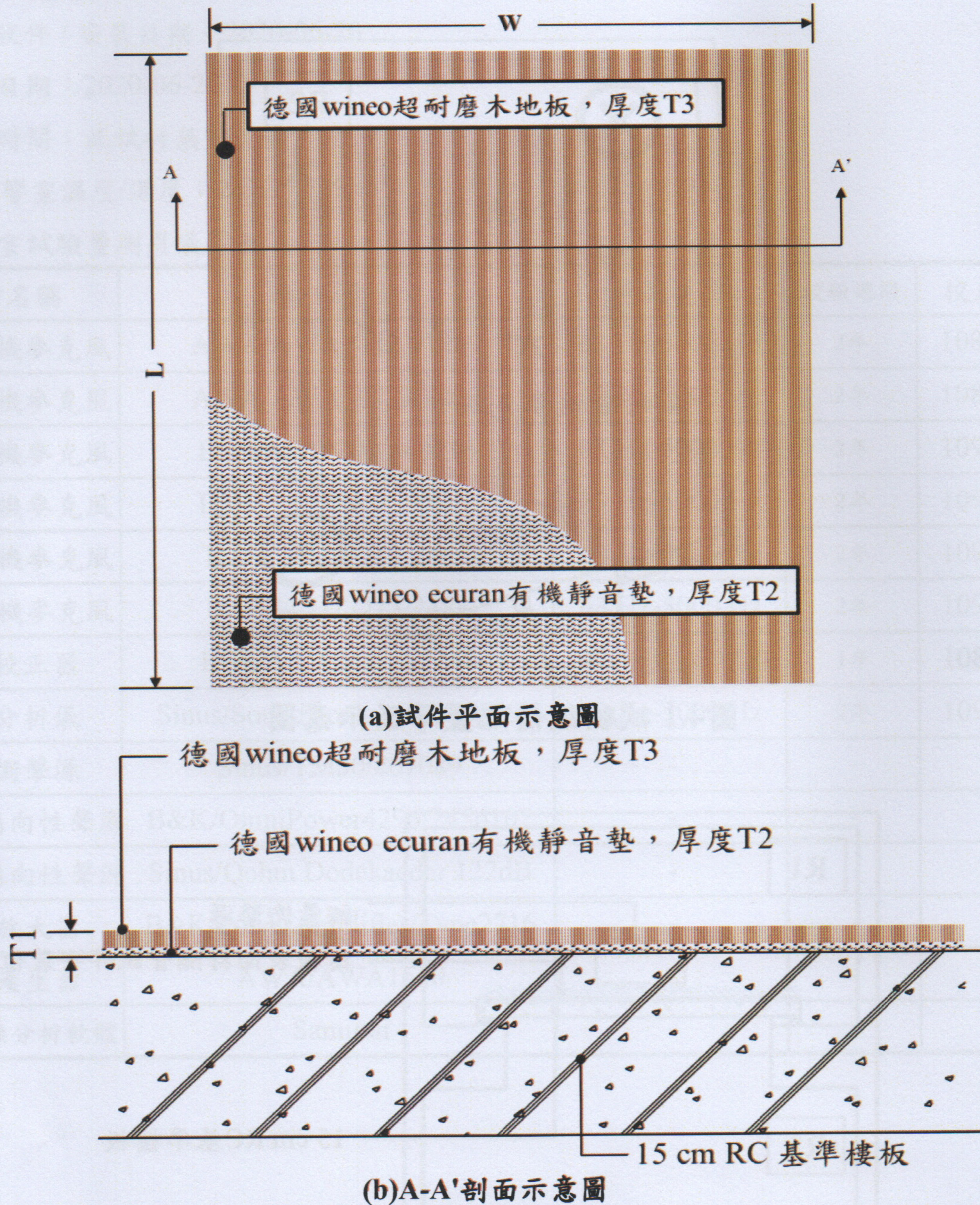
圖5.1 試件平面、剖面示意圖
